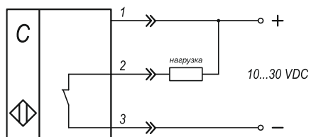
Рисунок 19 – Схема подключения NC датчиков NPN-типа
