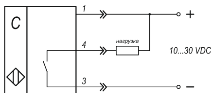
Рисунок 18 – Схема подключения NO датчиков NPN-типа
